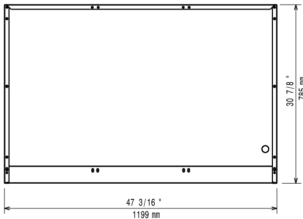
Felülnézet
